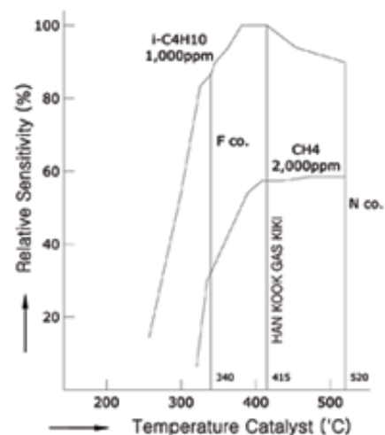
Sl.3) Karakteristike krive GASA
