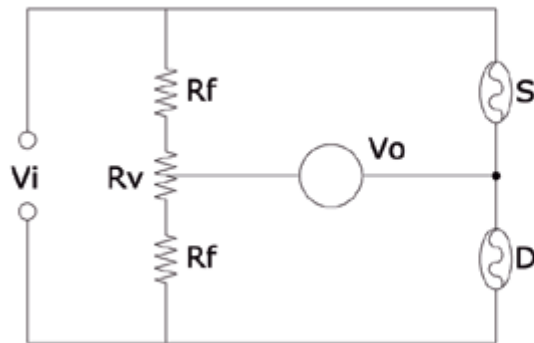
(Sl.2.) Tipično premosteno kolo
